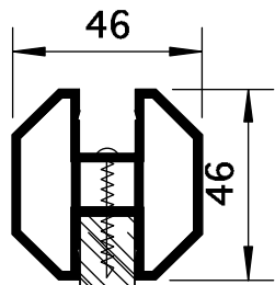
aluminium stabilisatieprofiel
