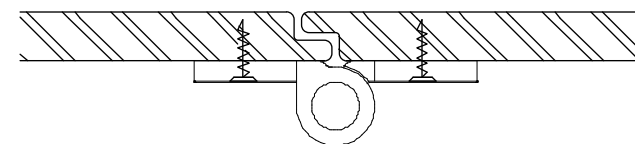
scharnier
